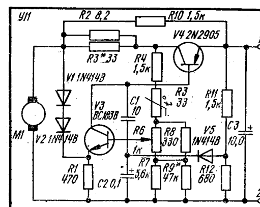
Принципиальная электрическая схема комплекса «Вега-117-стерео»:
